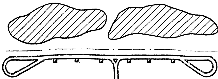
Рис.5. Подготовка полевым штреком с рудоспусками.
