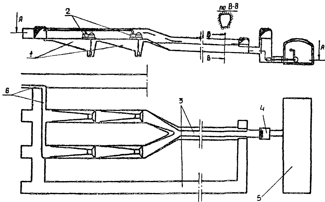
Рис.17. Схема водоотливного комплекса с насосной камерой заглубленного типа: 1- водоотстойники, 2 - flameвые насосы, 3 - водосборники, 4 - приёмный колодец, 5 - насосная камера.
