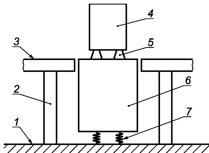
1 — грунтовое основание; 2 — стойка; 3 — пол лаборатории; 4 — испытуемое оборудование a ; 5 — жесткие опоры для установки испытуемого оборудования на фундамент b ; 6 — жесткий и массивный испытательный стенд c ; 7 — упругое опирание испытательного стенда на грунтовое основание d
