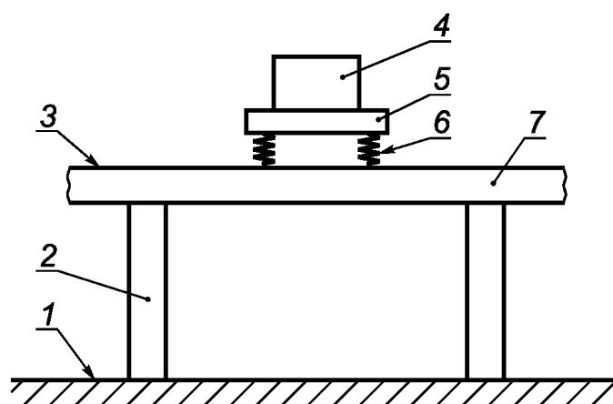
1 — грунтовое основание; 2 — стойка; 3 — пол лаборатории; 4 — испытуемое оборудование a ; 5 — крепежное приспособление; 6 — упругие опоры для установки испытуемого оборудования на фундамент b ; 7 — фундамент c
