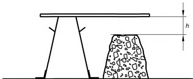
Рисунок 1 — Измерение осадки
