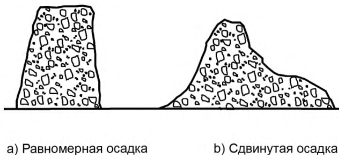
Рисунок 2 — Формы осадки
