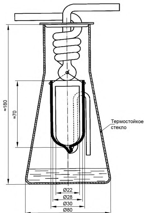
Рисунок 1 — Экстракционный аппарат
