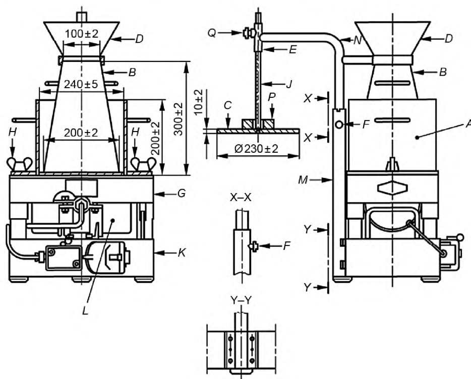
A — емкость; B — форма; C — прозрачный диск; D — воронка; E — направляющая муфта; F — винт; G — виброплощадка; H — винт барашковый; J — стержень с измерительной шкалой; K — полое основание; L — вибрирующий элемент; M — держатель; N — поворотный кронштейн; P — пригруз; Q — винт; Y-Y — деталь; X-X — деталь
