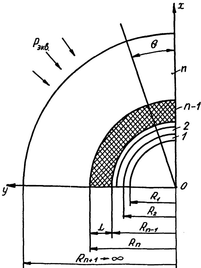
Рис. 2.1. Расчетная схема крепи горизонтальной выработки круглого сечения в упрочненном массиве: 1, 2 - слой крепи, которая в общем случае может быть многослойной; n-1 - зона упрочненных пород; R_n - массив пород; R_1, \dots, R_{n-1}, R_{n+1} - внутренние радиусы соответствующих слоев крепи; \theta - полярный угол; L - толщина упрочненных пород
