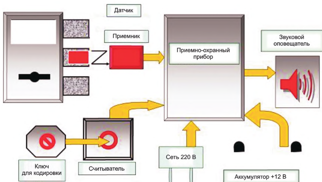
Рисунок Г.1 — Блок-схема системы раннего реагирования
