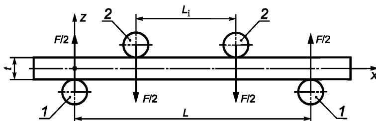
Рисунок 1 — Схема нагружения при испытании на трехточечный изгиб
