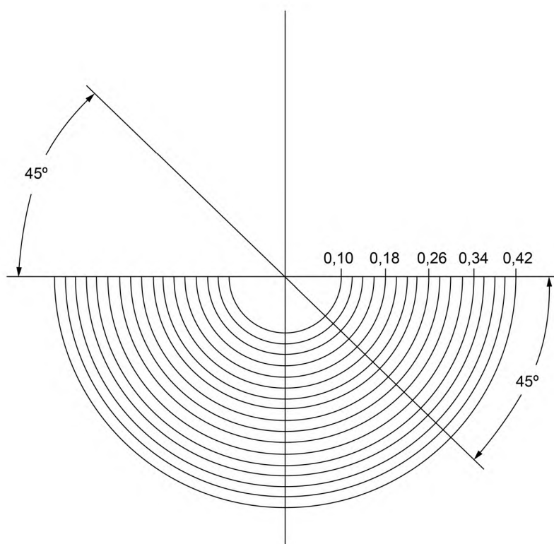
Рисунок А.1 — Пример прозрачного шаблона для увеличения 100×
