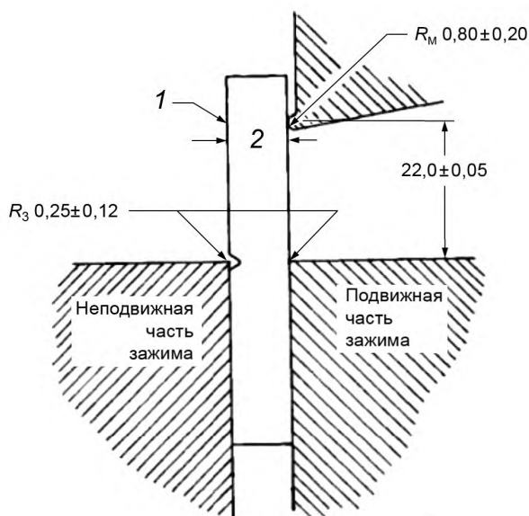
1 — образец; 2 — толщина образца; R_3 — радиус верхнего края зажима; R_M — радиус лезвия маятника
