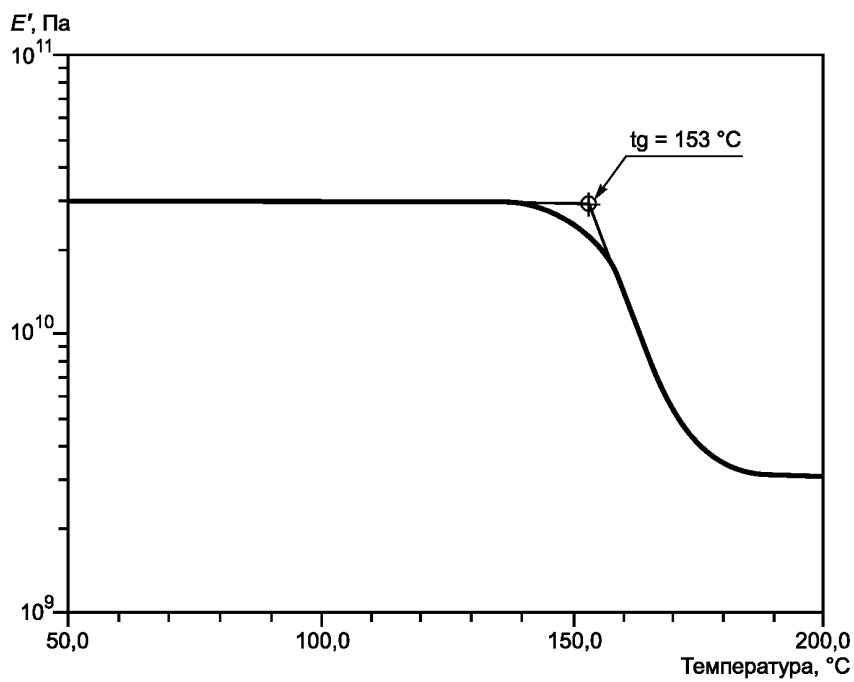
Рисунок X1.2 — Пример определения температуры стеклования T_g
