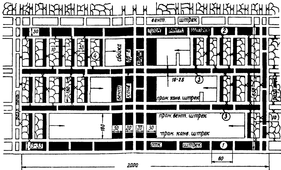
— целики, соседних выемочных участков — целики, теряемые полностью Схема 4. Система разработки длинными столбами по простираанию с оставлением целиков в выработанном пространстве.
