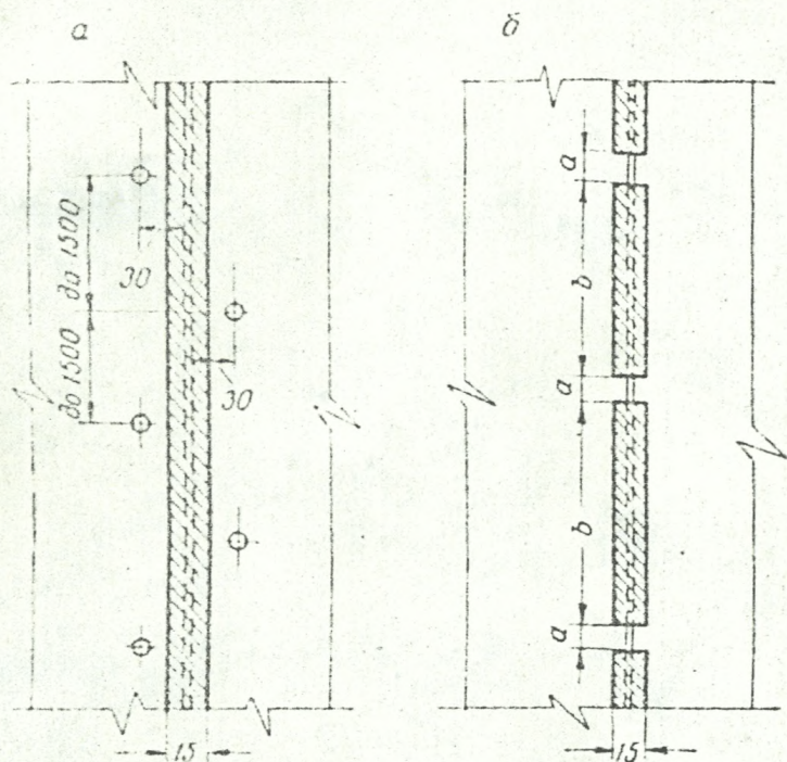
Рис. 8. Схема обработки трещин: а — для глубинного иньектора; б — для поверхностного иньектора (обработанные участки трещины заштрихованы).
