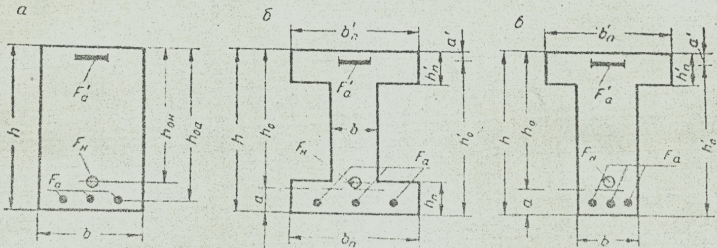
Рис. 6. Геометрические характеристики сечений: а — прямоугольного; б — двутаврового; в — гравового.
