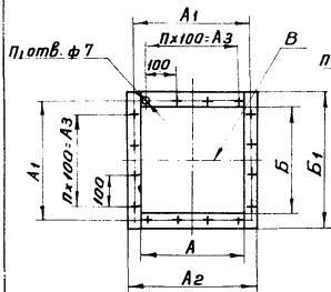
Фланец выходной вентиляторов н 3,15; 4; 5; 6,3
