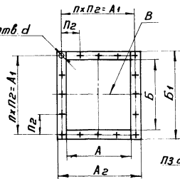
Фланец выходной вентиляторов н 2,5; 8
