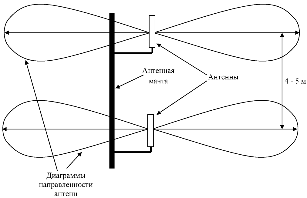
Рис. Г2 «Разнос» антенн по вертикали
