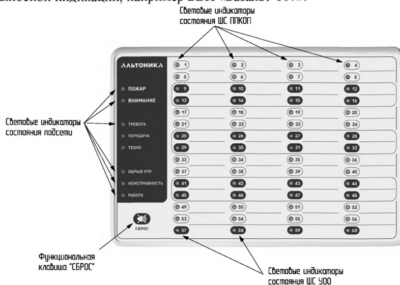
Рис. 148 Внешний вид БВИ «Базальт-607»
