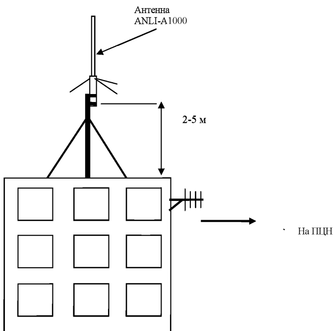
Рис. 26 Показана взаимная экранировка стен здания антенн БРР
