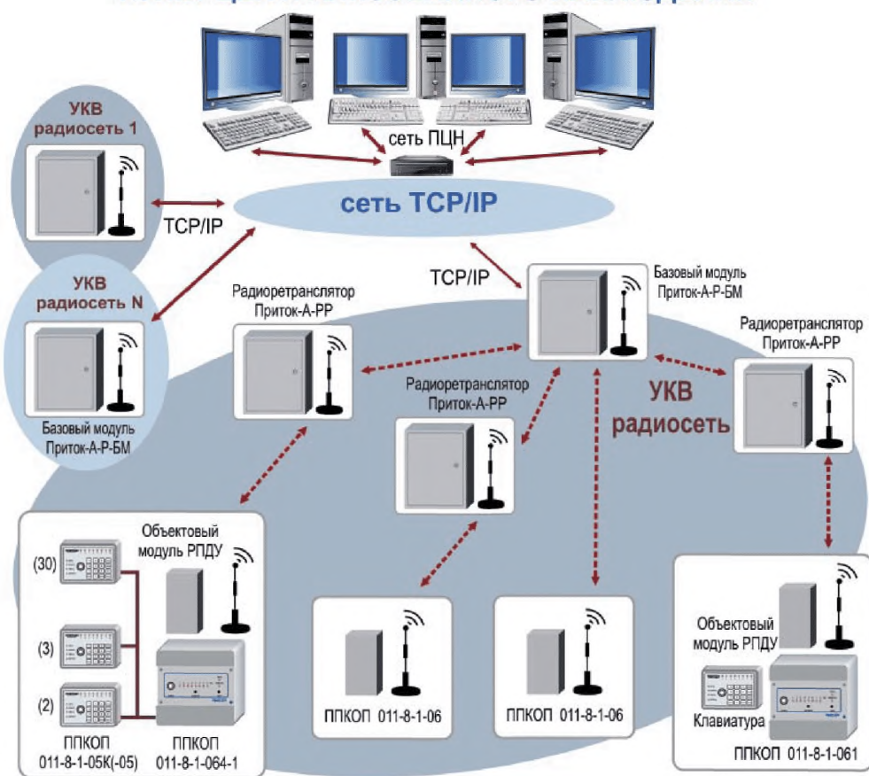
Рис. 74 Структурная схема «Приток-А-Р»
