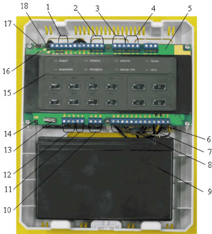
Рис. 147 Внешний вид УОО «Базальт-281» со снятой крышкой
