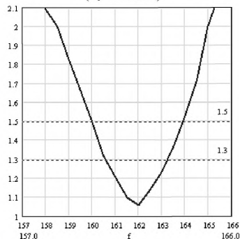
График КСВ А-1000 MV1 (F 0 =162МГц)
