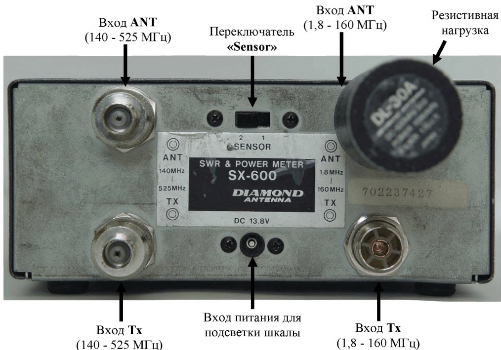
Рис. А12 Задняя панель КСВ-метра DIAMOND SX-600
