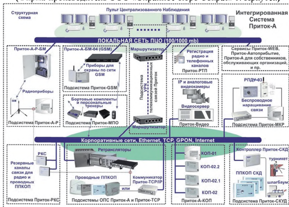
Рис. 73 Структурная схема «Приток-А»
