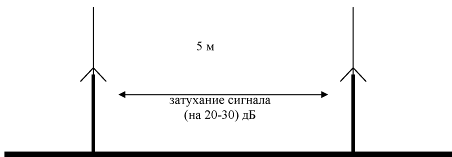
Рис. Г3 «Разнос» антенн по горизонту
