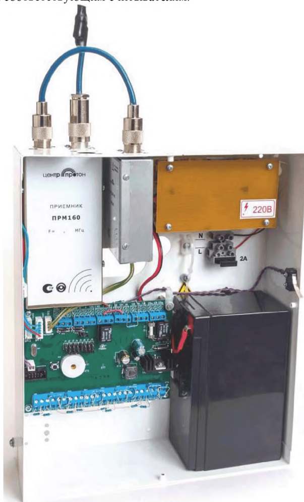
Рис. 124 Внешний вид ППКОП «Протон-16», «Протон-8»
