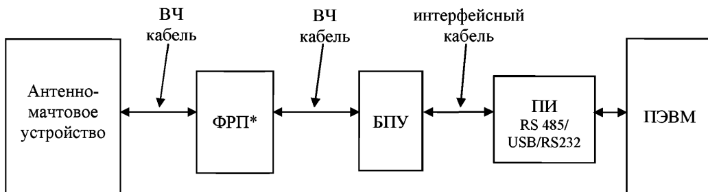
Рис. 23 Схема ПЦН РСПИ «Струна-5»
