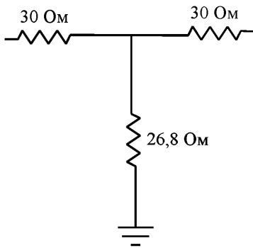
Рис. А14 (ослабитель на 12 дБ)
