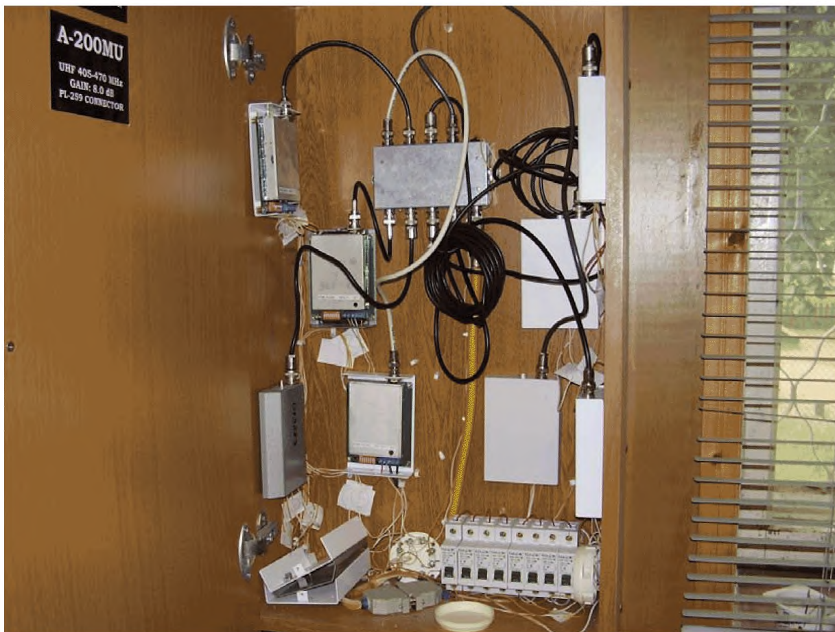
Рис. В5 Скручивать кабель в бухту недопустимо
