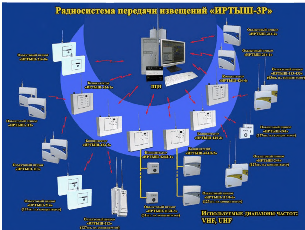
Рис. 56 Структурная схема РСПИ «Иртыш-3Р»
