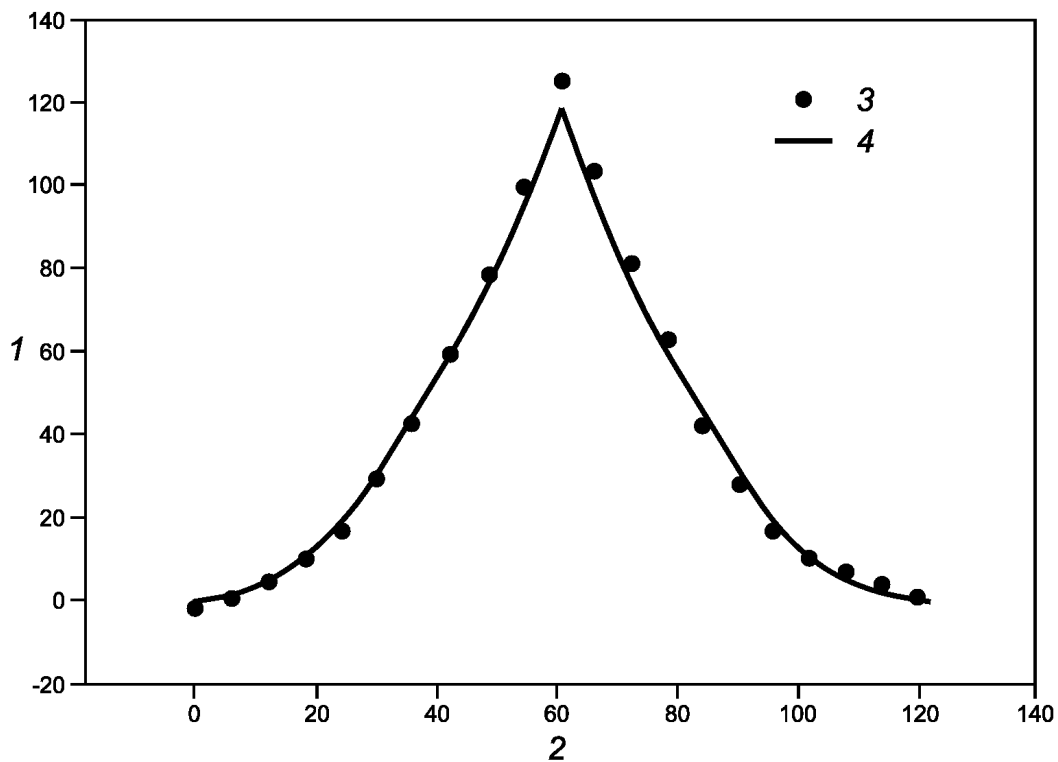
1 — измерение; 2 — время; 3 — экспериментальные данные; 4 — прогноз модели
