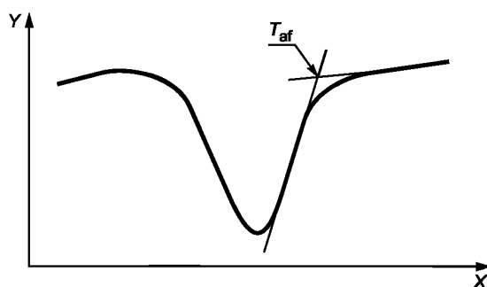
Рисунок 2 — Кривая дифференцирующей сканирующей калориметрии
