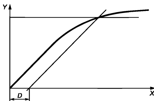
Рисунок 4 — График жесткости при изгибе
