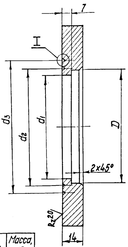
Размеры в мм
