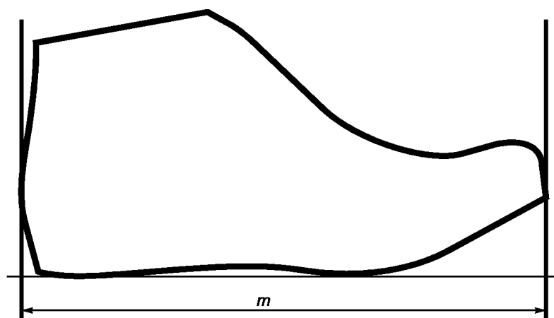
Рисунок А.9 — Мерочная длина колодки
