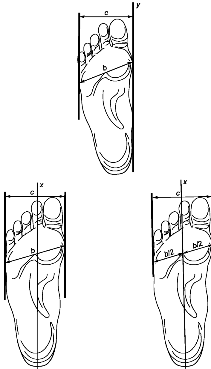
a — Мерочная длина стопы (метод 1) b — Мерочная длина стопы (методы 2а и 2б) b — ширина следа в носочно-пучковой части стопы; c — мерочная ширина стопы; x — центральная линия стопы; y — касательная к внутренней стороны стопы
