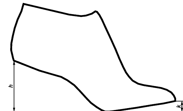
Рисунок А.7 — Линия контура следа колодки
