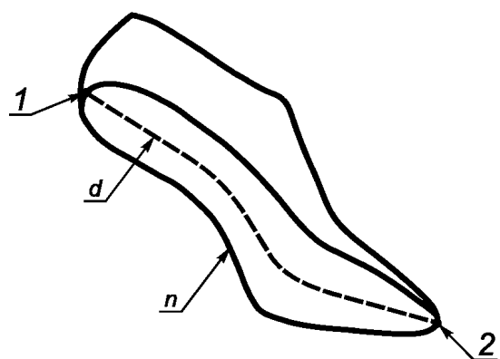
а – Центральная линия следа колодки (метод 1)
