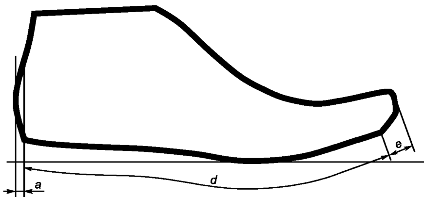
a — пяточный изгиб колодки; d — длина следа колодки; e — нависающая носочная часть колодки Рисунок А.6 — Длина колодки
