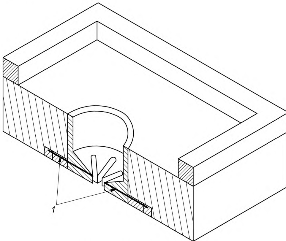
1 — проволочные электроды (диаметром 1,6 мм)
