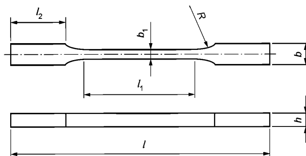
l — длина образца; l_1 — длина рабочей части образца; l_2 — длина захватов; b — ширина образца; b_1 — ширина рабочей части образца; h — толщина образца; R — радиус закругления
