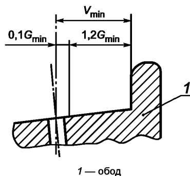
Рисунок 9 — Расположение отверстия для вентиля камерной шины
