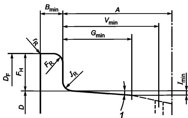
Рисунок 5 — Сечение посадочной полки
