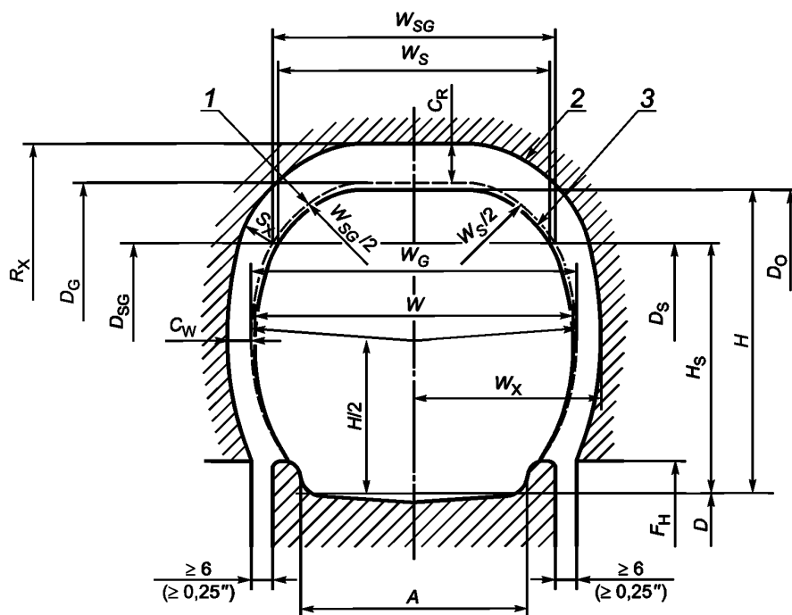
Рисунок 2 — Допуски на увеличение и на зазоры
