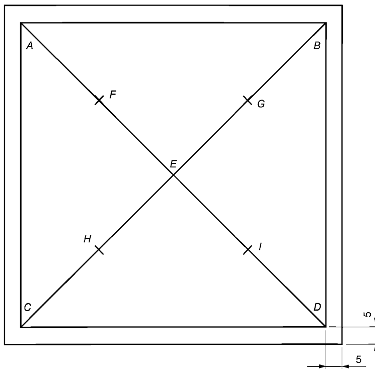
Рисунок 1 — Разметка образца для испытания
