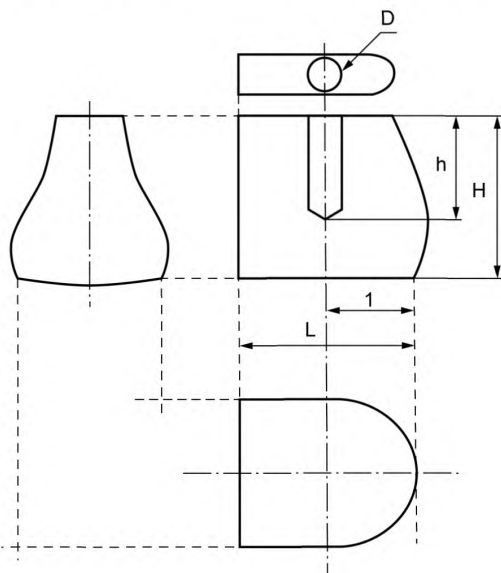
Рисунок 1 — Испытательное приспособление для определения энергии сжатия
