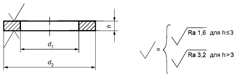
Рисунок 1 — Размеры
