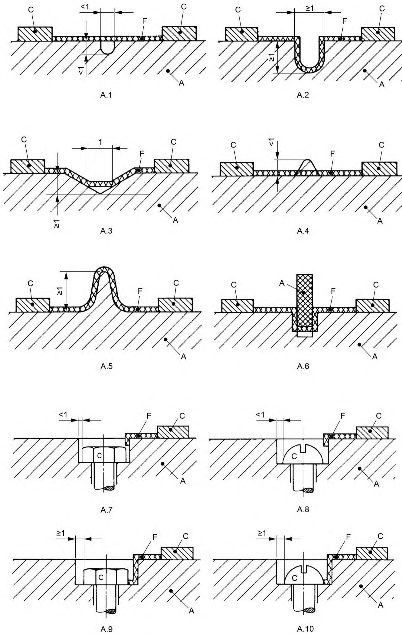
Рисунки А.1—А.10 — Примеры определения расстояний утечки
