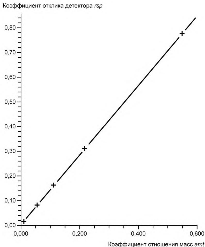
Рисунок 3 — Типовая калибровочная кривая для бензола
