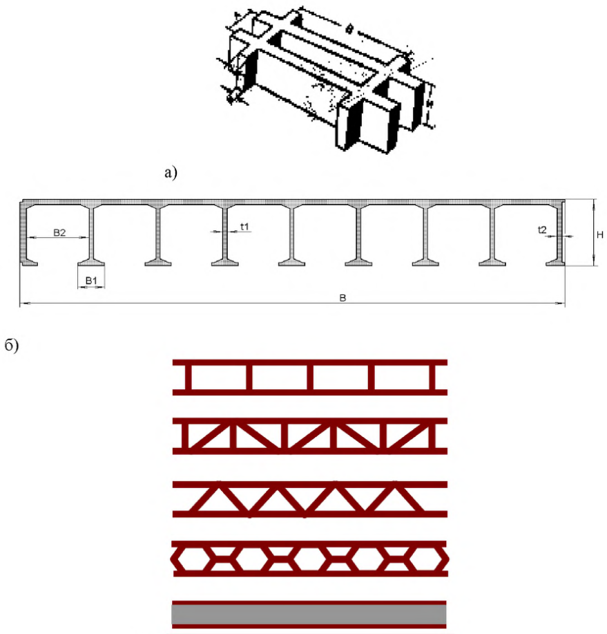
Рисунок 1 – Примеры поперечных сечений секций настилов
