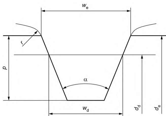
Рисунок 3 — Канавка испытательного шкива
