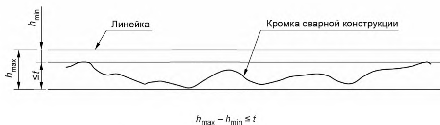
Рисунок 6 — Испытание на прямолинейность
