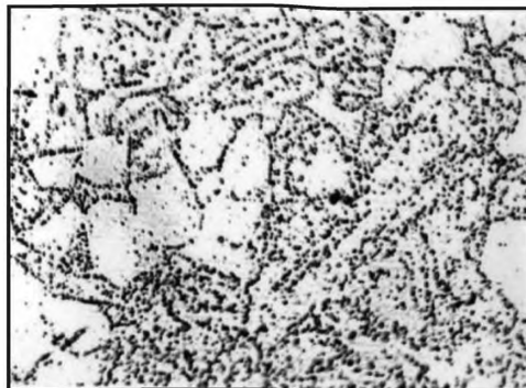
Балл 2, 500 x , электролитическое травление
