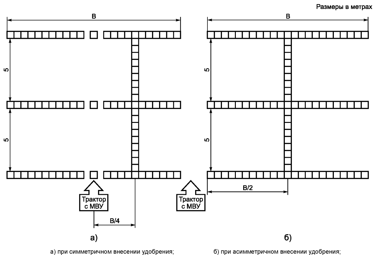
Рисунок 1 — Схема размещения контейнеров при определении показателей качества выполнения технологического процесса
