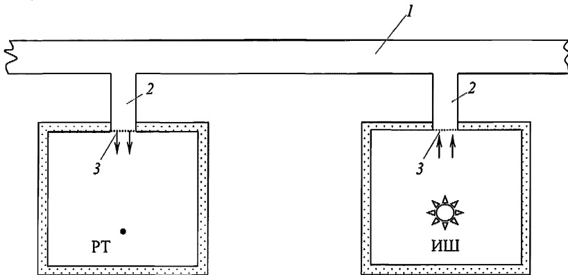
1 – вентиляционный канал; 2 – ответвления от вентиляционного канала к помещениям; 3 – концевые воздухораспределительные устройства (решетки, плафоны и т.п.); ИШ – источник шума; РТ – расчетная точка
