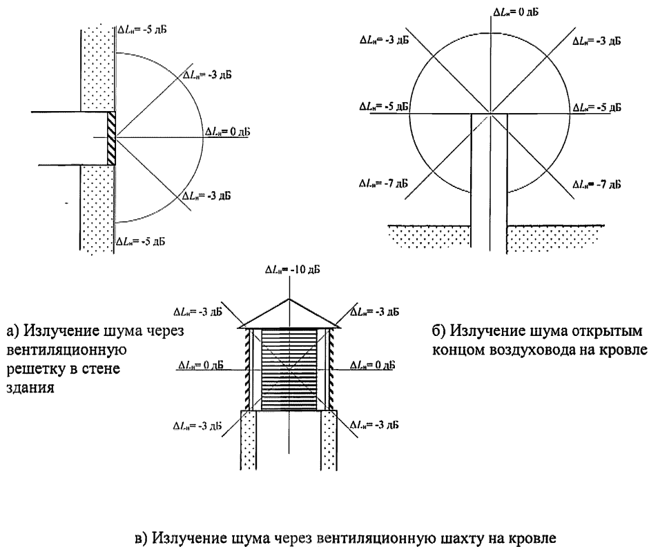
Рисунок 8.3 – Показатель направленности излучения шума через отверстия вентиляционных решеток, воздуховодов, шахт и подобных элементов
