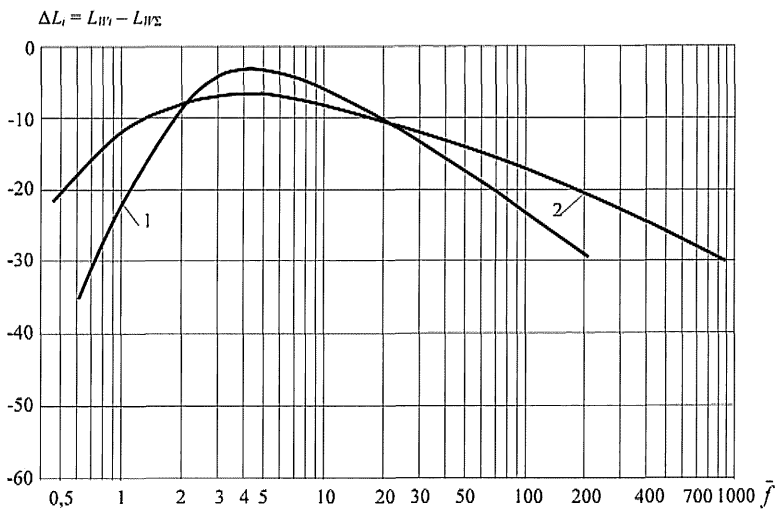
Рисунок 6.13 – Безразмерные частотные характеристики воздухораспределителей
