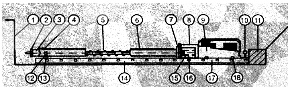
Рисунок 5 – Установка горизонтального шнекового бурения
