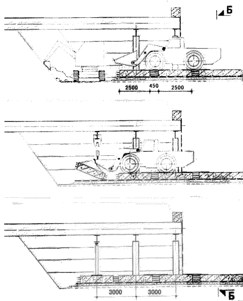
Рисунок 16 – Технологическая схема сооружения тоннеля под защитой экрана из труб
