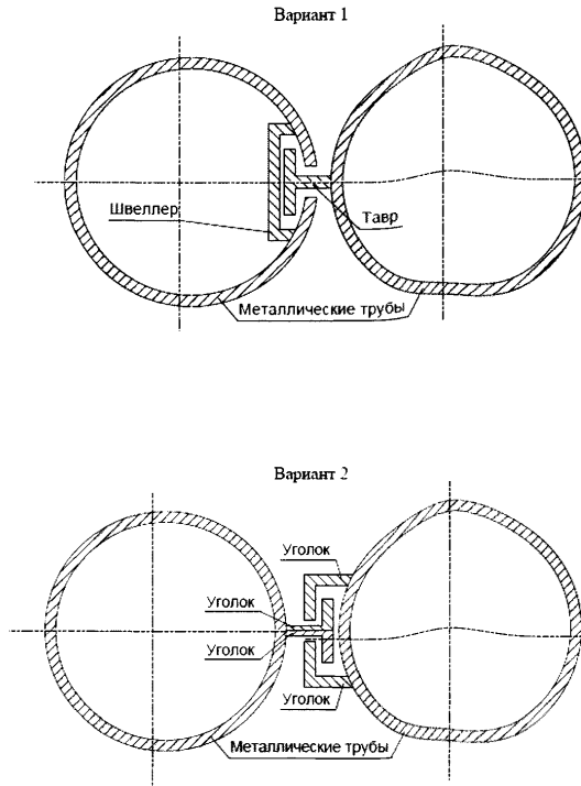
Рисунок 1 – Схемы фиксирующих устройств труб экрана
