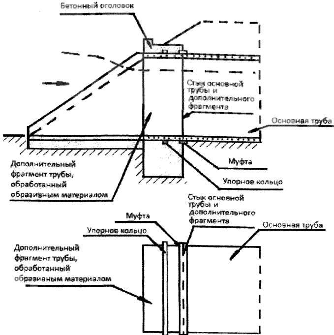
Рисунок 18 – Конструкция оголовка композитной водопропускной трубы
