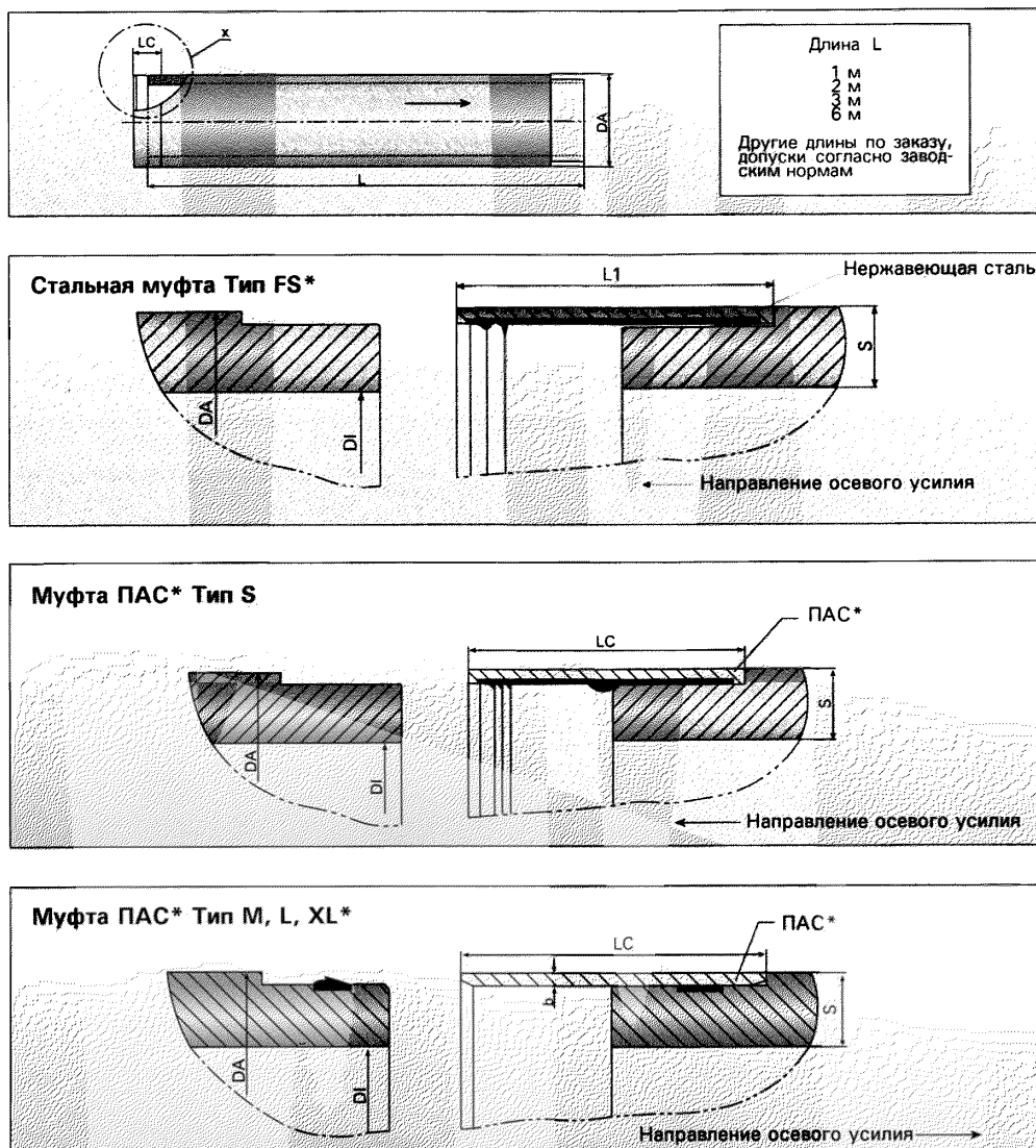
Рисунок 4 - Соединительные муфты
