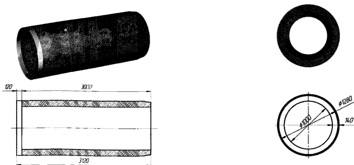
Рисунок 2 – Звено трубы для бестраншейной прокладки
