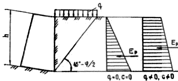
Рисунок Г.2 – Схема к расчету пассивного давления грунта на вертикальную гладкую стенку
