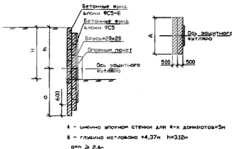
Рисунок Г.1 – Схема типовой упорной стенки Тип IV
