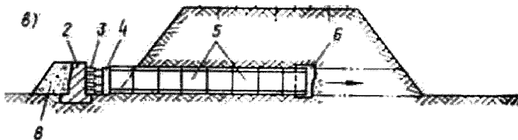
1 – насыпь; 2 – железобетонный упор; 3 – домкратная установка; 4 – распределительное кольцо; 5 – продавливаемые секции; 6 – ножевая часть щита.
