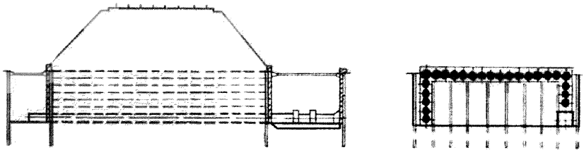
Рисунок 15 – Устройство вертикальных рядов экрана из труб
