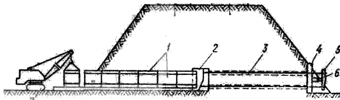
1 – секции обделки тоннеля; 2 – ножевая секция; 3 – тросы; 4 – упорная стенка; 5 – траверса; 6 – домкрат.
