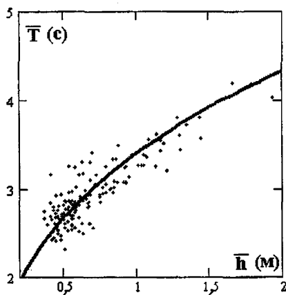
Рис. 5.7 Соотношение между высотами и периодами волн на Каспийском море
