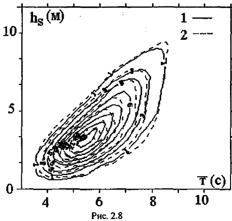
Рис. 2.8 Совместные распределения значительных высот и средних периодов волн. 1—инструментальные измерения, 2—модельные расчеты
