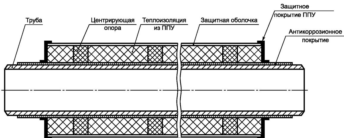
Рисунок 6.1 — Конструкция трубы в теплоизоляции
