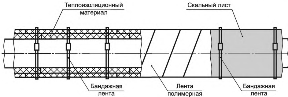
Рисунок 6.7 — Конструкция трубы в теплоизоляции с использованием скорлуп
