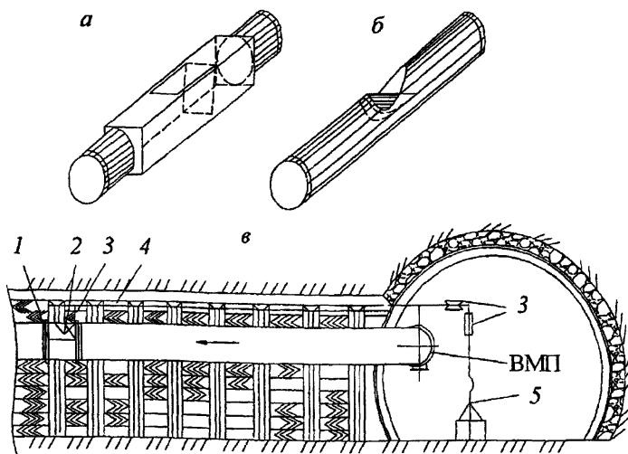
Рис. 1. Устройство для разгазирования тупиковых горных выработок: а, б - схемы устройства; в - схема установки; 1 - патрубкок; 2 - клапан; 3 - ролики; 4 - трос; 5 - ручная (электрическая) лебедка
