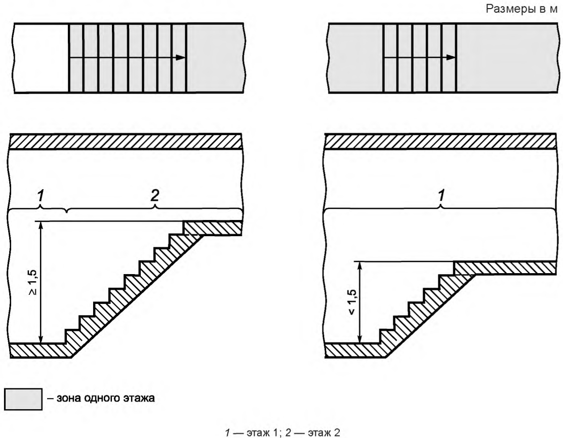
Рисунок В.3 — Пример уровней этажей
