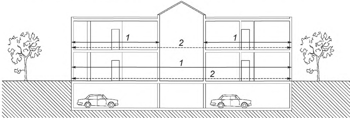
Рисунок В.1 — Пример площади этажа и общей площади этажа, включая атриум
