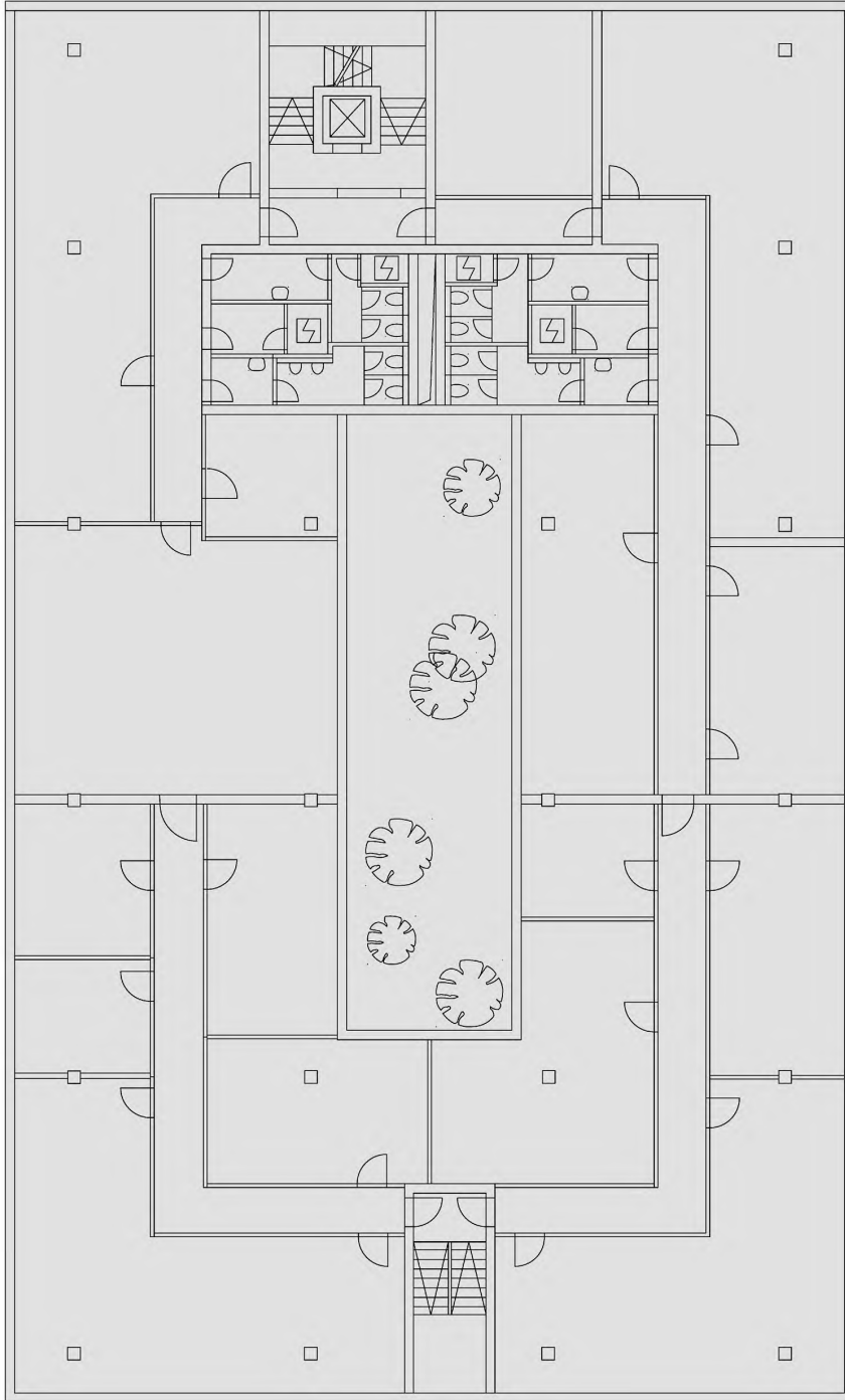
Рисунок 5 — План этажа
