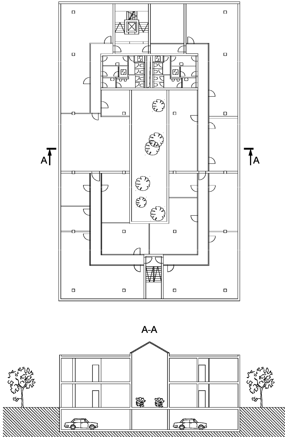
Рисунок 4 — Постажный план здания и план верхнего этажа
