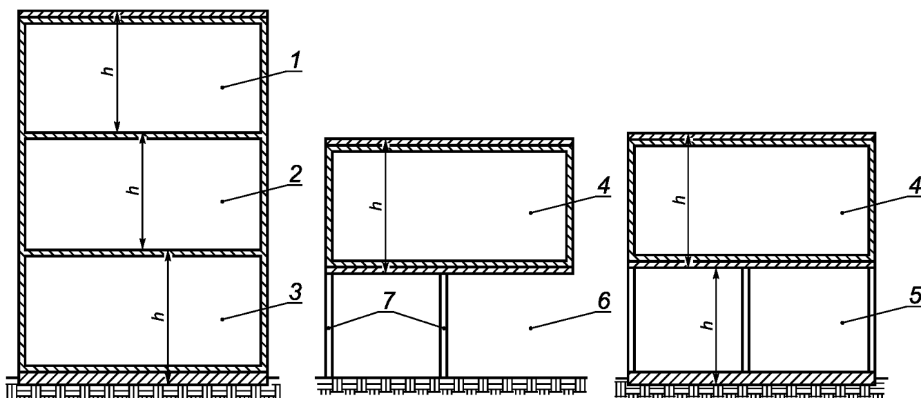
Рисунок 1 — Измеряемые размеры помещения
