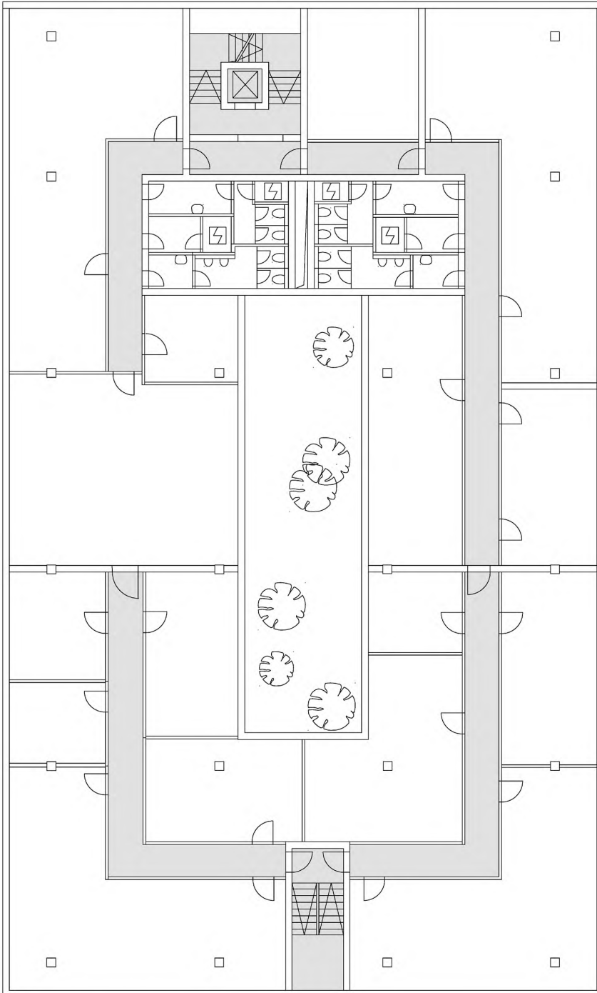
Рисунок 15 — План этажа с указанием зон перемещения людей
