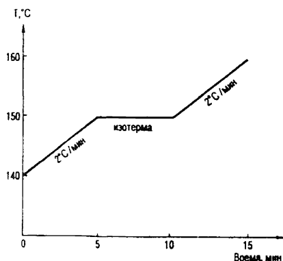
Рис. 8. График программирования температуры.
