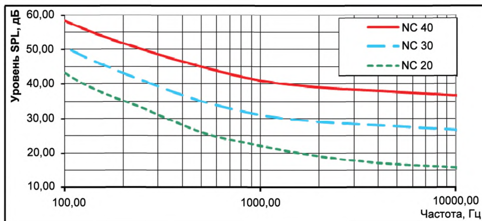
Рисунок 4 — Спектральная плотность окружающего шума
