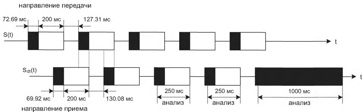
Рисунок 13 — Тестовые сигналы для определения диапазона затухания в направлении приема во время одновременного разговора
