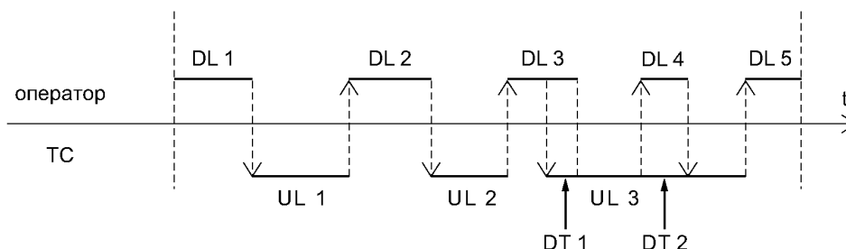
Рисунок 15 — Последовательность проигрывания записей.
