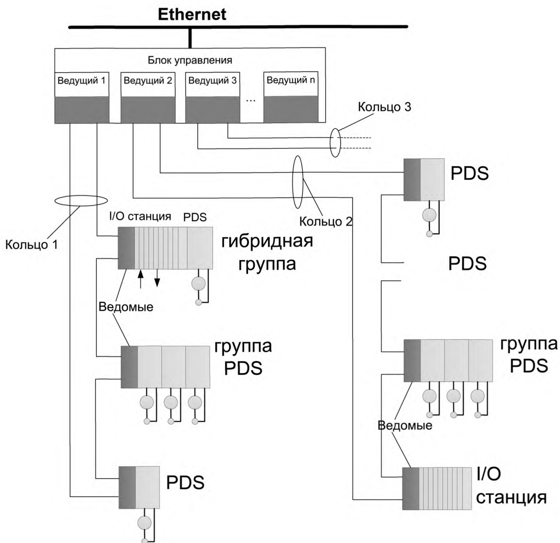
Рисунок А.2 — Пример топологии
