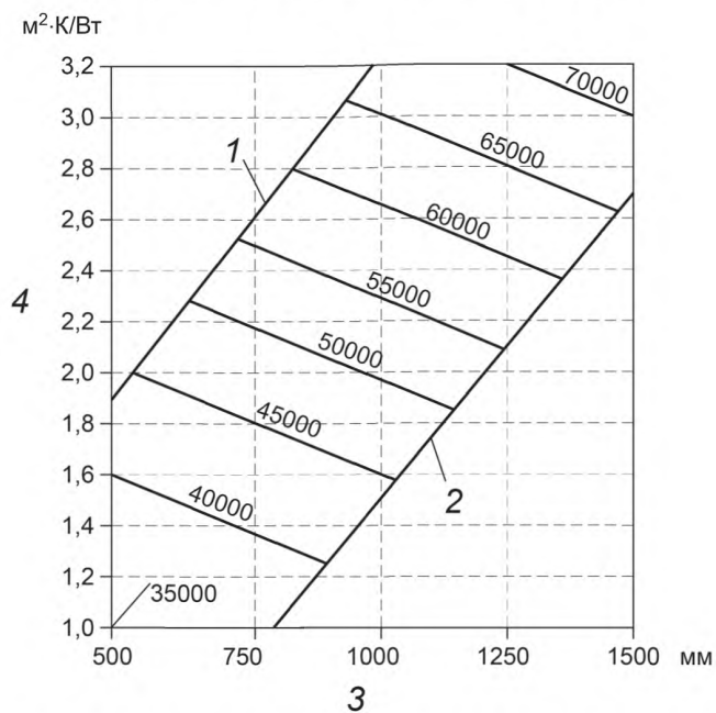
1 — минимальная b_{gc} ; 2 — минимальная R_{gc} ; 3 — ширина теплоизоляции грунта b_{gc} ; 4 — сопротивление теплопередаче теплоизоляции грунта на углах R_{gc}
