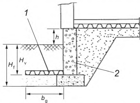
а) Ленточный фундамент с теплоизоляцией грунта
