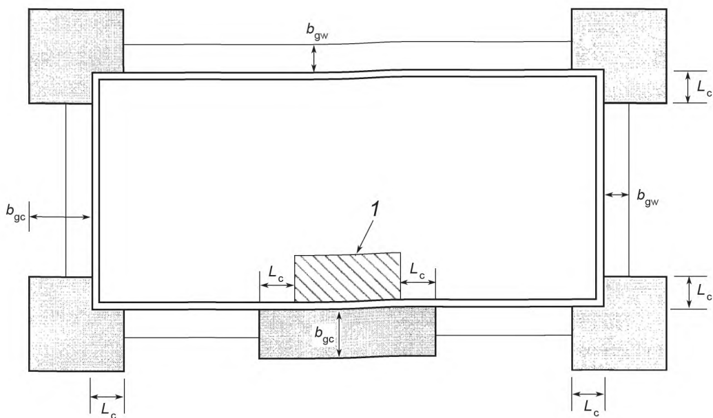
1 — ограниченная неотапливаемая часть (кладовая, крыльцо и т.п.)
