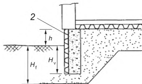
д) Ленточный фундамент с вертикальной теплоизоляцией
