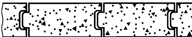
ф) Бетонные шпунтовые сваи, образующие стенку в грунте
