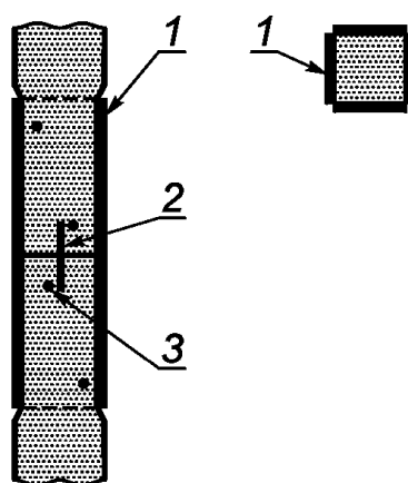
Рисунок А.8 — Пример комбинированной сваи
