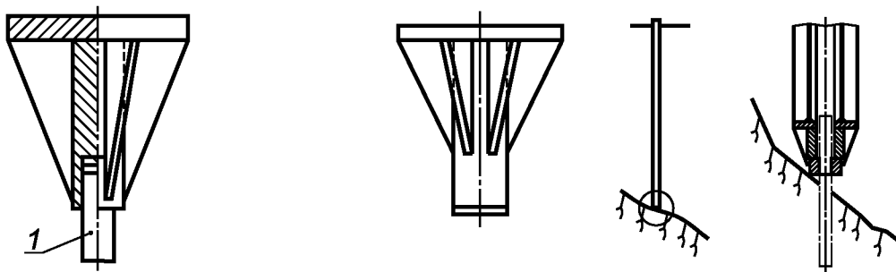
д) Скальный башмак для наклонных скальных поверхностей
