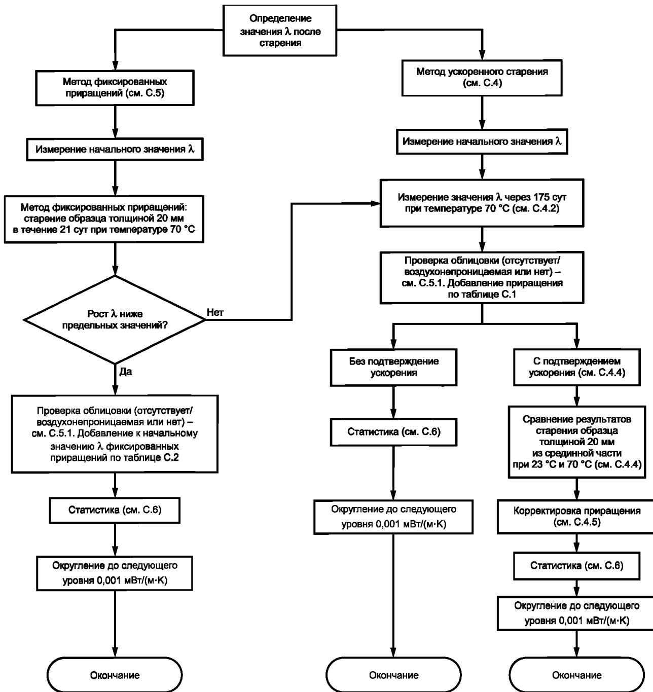
Рисунок С.1— Блок-схема альтернативных методов старения
