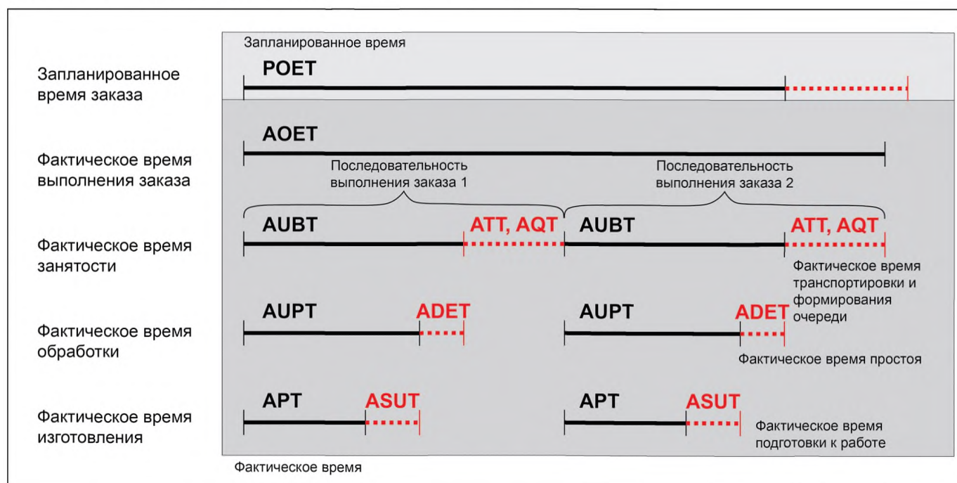
Рисунок С.2 — Временной график выполнения производственных заказов
