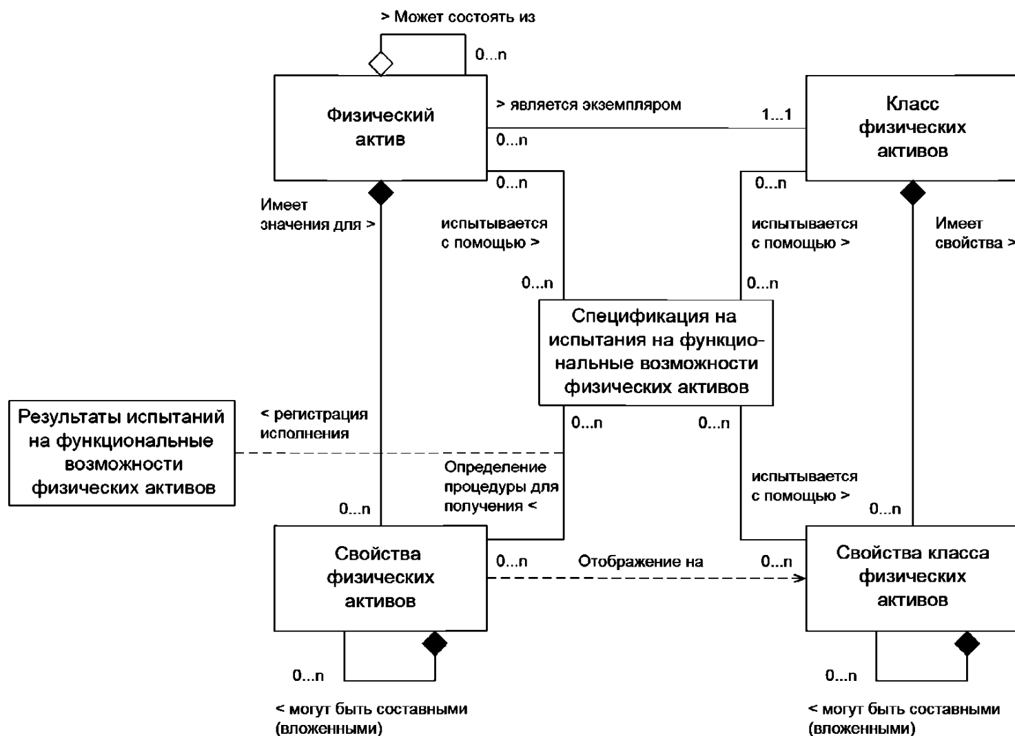
Рисунок В.3 — Модель физических активов [МЭК 62264-2]
