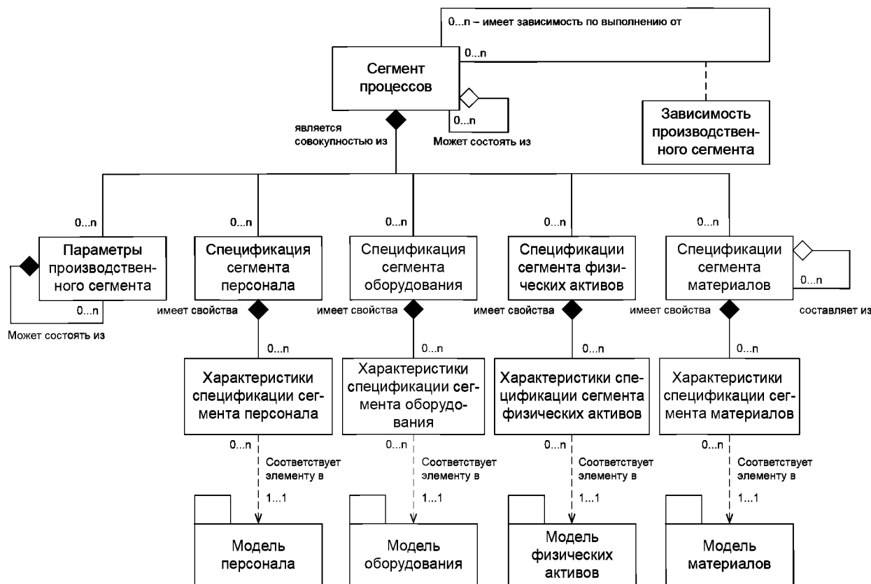
Рисунок А.6 — Модель производственного сегмента [МЭК 62264-2]
