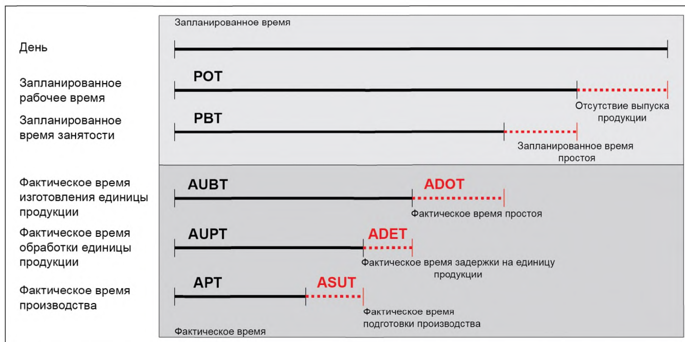
Рисунок С.1 — Временной график использования единиц технологического оборудования в процессе производства
