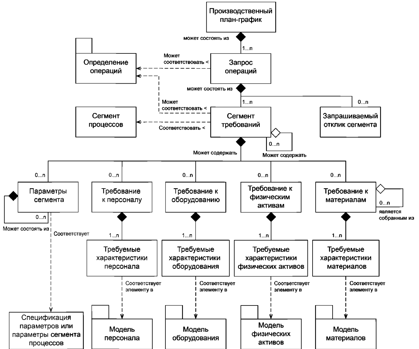
Рисунок А.8 — Модель производственного план-графика [МЭК 62264-2]
