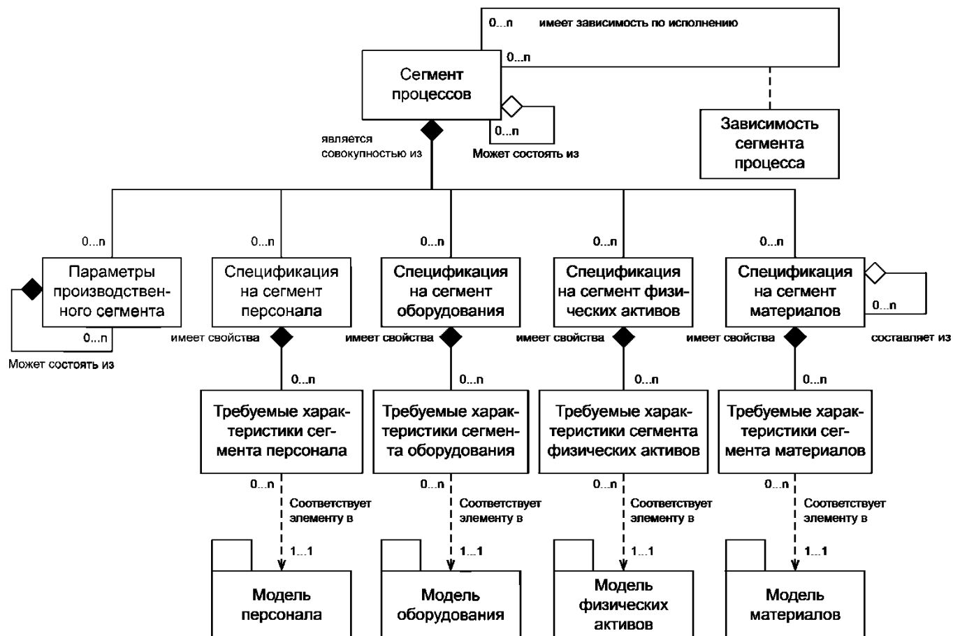
Рисунок В.5 — Модель производственного сегмента [МЭК 62264-2]
