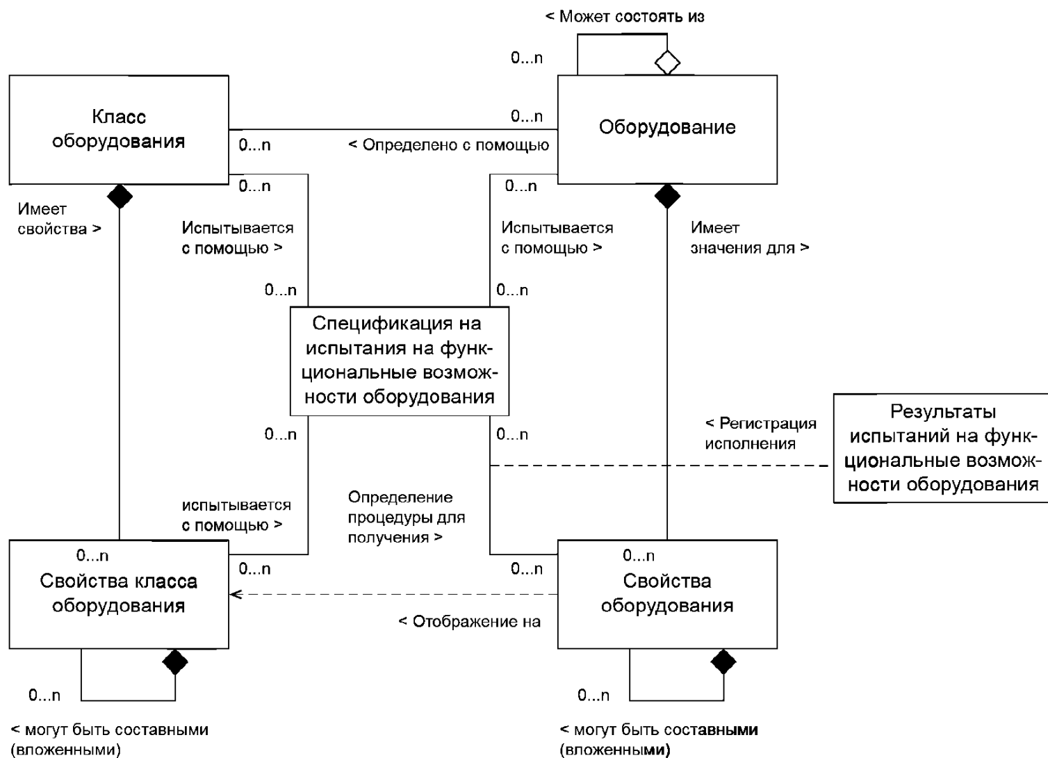
Рисунок В.2 — Ролевая модель оборудования [МЭК 62264-2]
