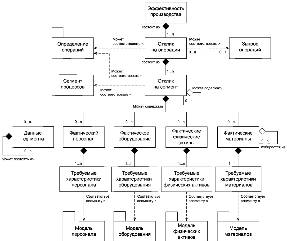
Рисунок A.9 — Модель эффективности производства [МЭК 62264-2]
