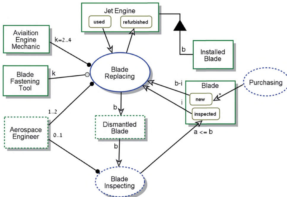
Рисунок 33, лист 1 — Диаграмма, иллюстрирующая кратность объекта: арифметические выражения и пример ограничений
