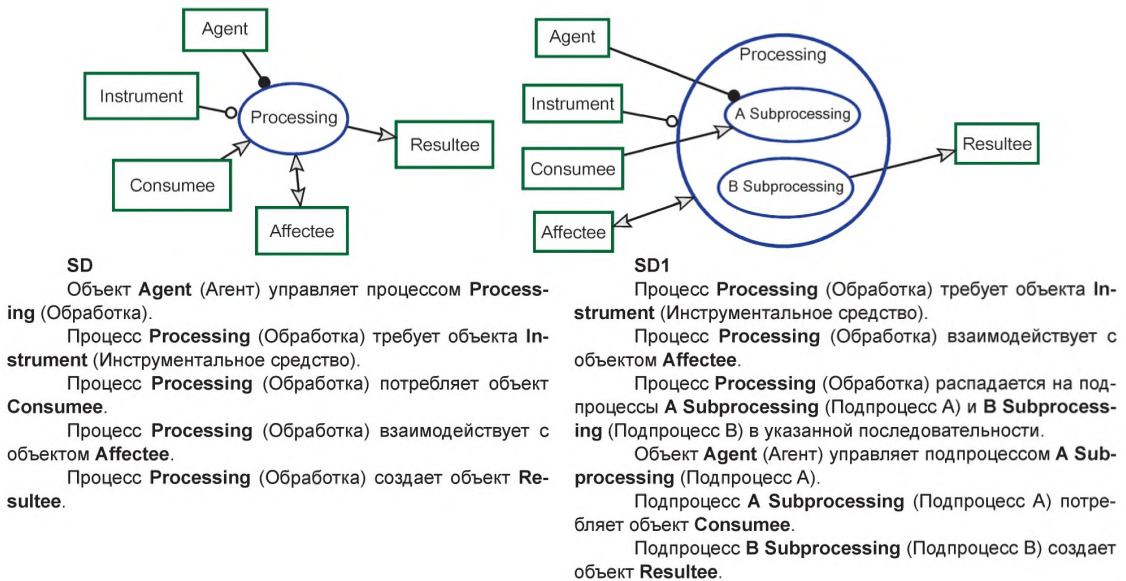
Рисунок 46 — Пример новой детализированной диаграммы
