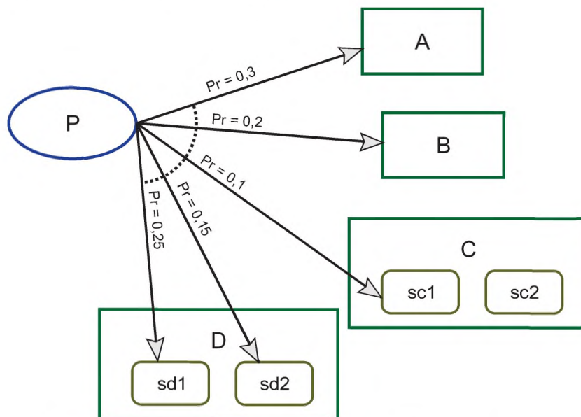
Рисунок 42, лист 1 — Объекты, имеющие или не имеющие определенных состояний, как источники и получатели вероятностной веерной связи
