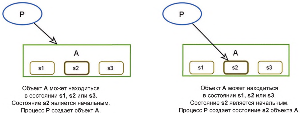
Рисунок 10 — Правильно (слева) и неправильно (справа) обозначенная результирующая связь с объектом, имеющим начальное состояние
