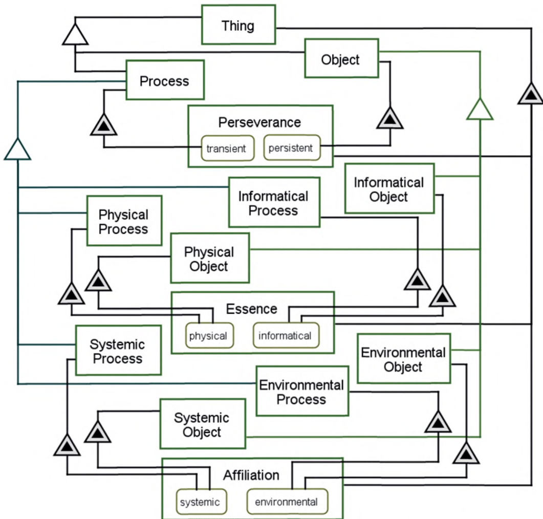
Рисунок С.9, лист 1 — Диаграмма ОРМ-модели общих свойств объекта Thing
