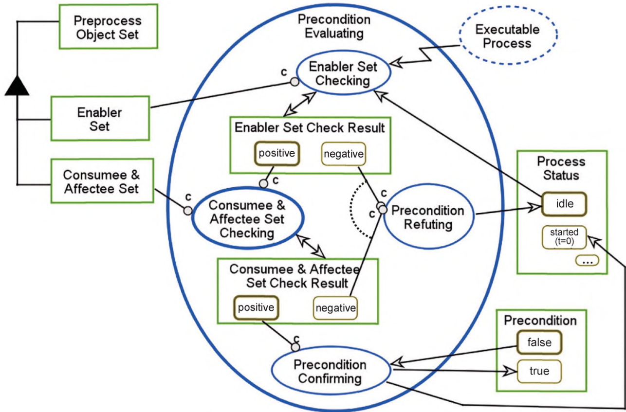
С.6.4 Детализированная диаграмма процесса Precondition Evaluating (диаграмма SD1.1.1)
