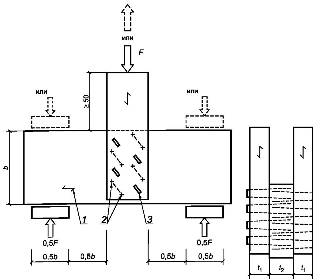
Рисунок 4 — Образец для испытания на одинарный сдвиг, нагруженный на растяжение или сжатие, со средним элементом, нагруженным поперек волокон (На рисунке 4 показано соединение с углом \alpha_{см} = 45^\circ .)
