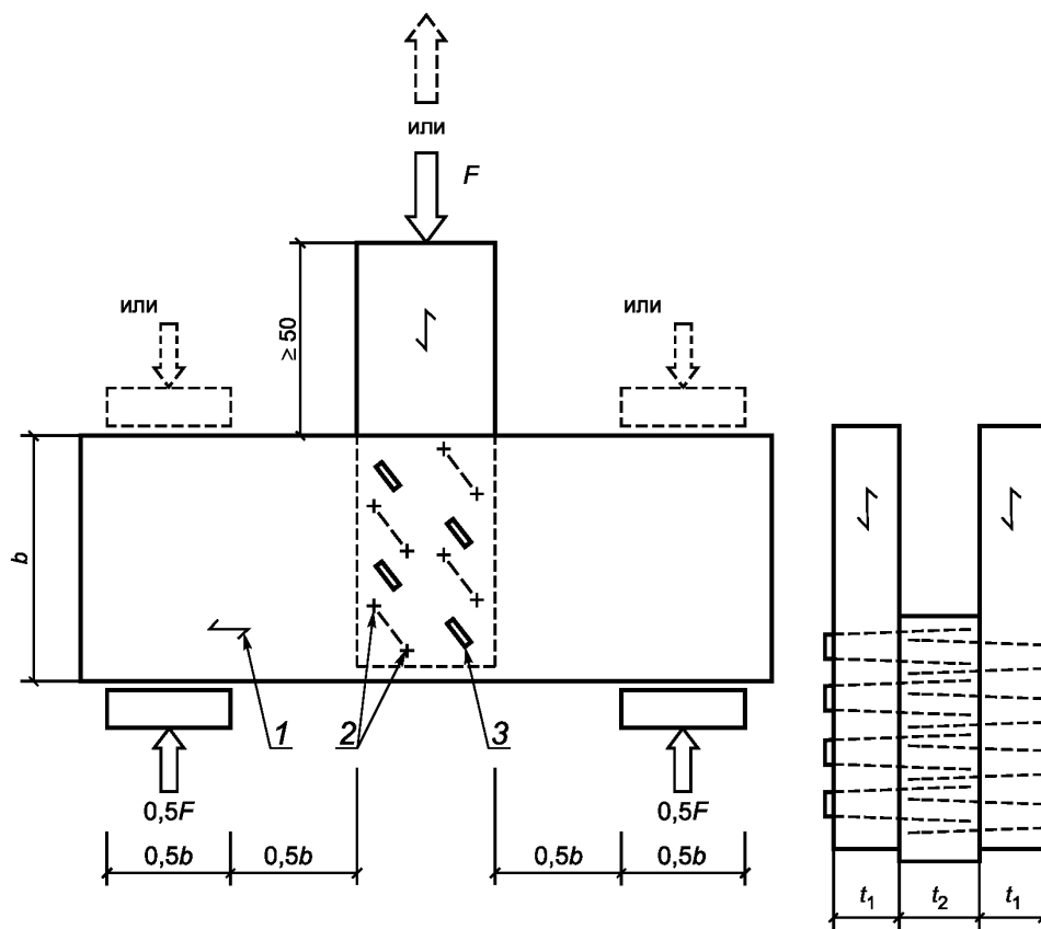
1 — направление волокон; 2 — острие скобы; 3 — перекладина скобы
