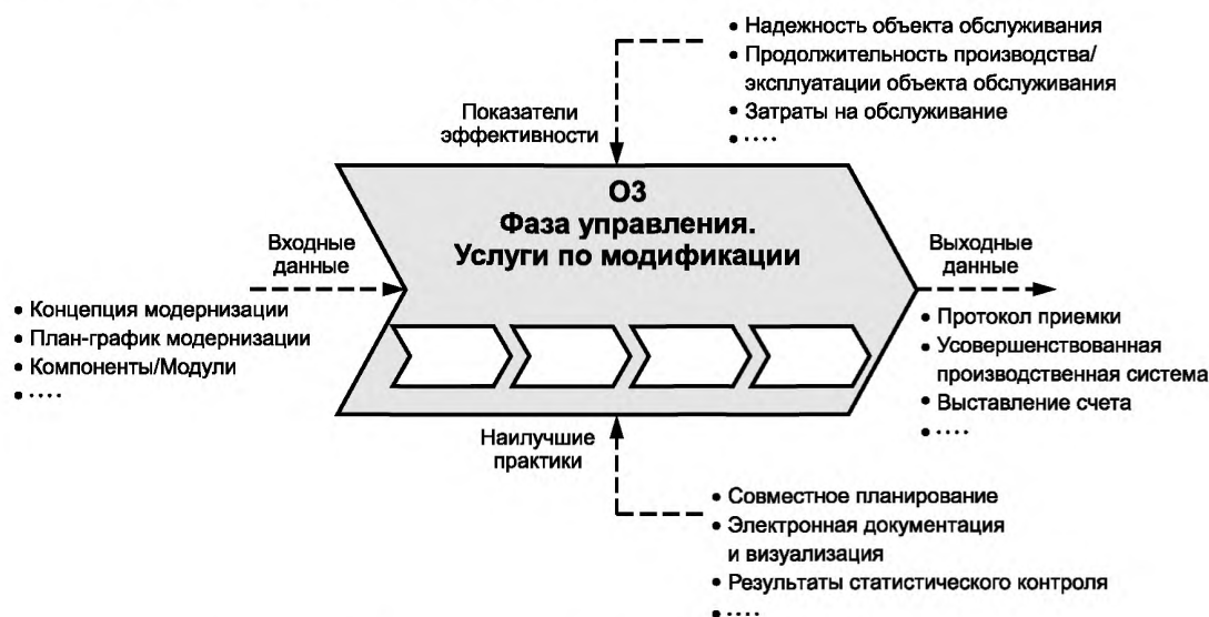
Рисунок 17 — Фаза управления. Услуги по модификации (O3)
