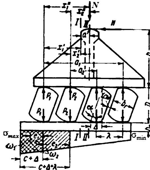
Рисунок 7.2.3 – Схема к расчету нижнего балансира и опорной плиты - моменты от нагрузок в сечениях балансира I и II
