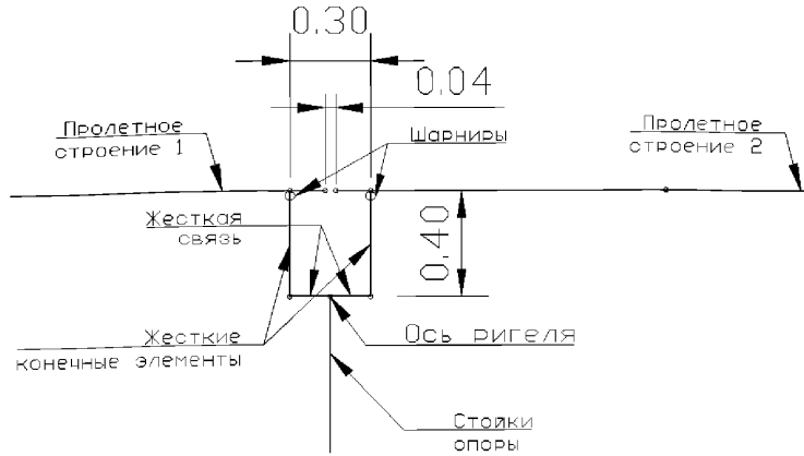
Рисунок Г.1.3 – Узел А
