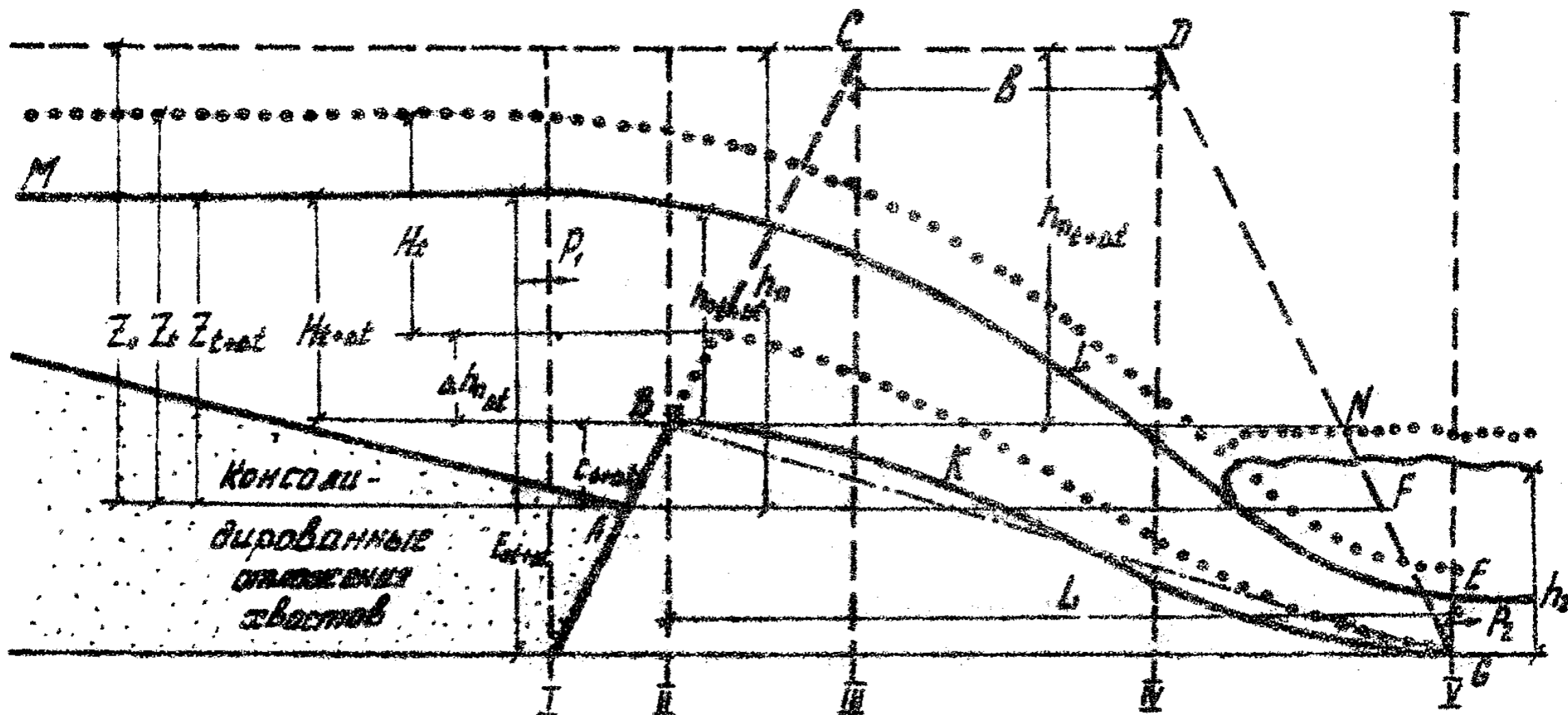
Рис. I. I. Схема развития плотины хвостокранника.
