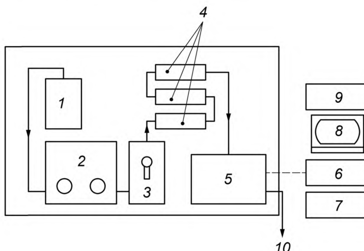
1 — резервуар для подвижной фазы; 2 — насосы; 3 — блок ввода пробы; 4 — хроматографические колонки; 5 — детектор; 6 — компьютер; 7 — устройство регистрации данных; 8 — экран; 9 — графопостроитель (плоттер); 10 — на слив
