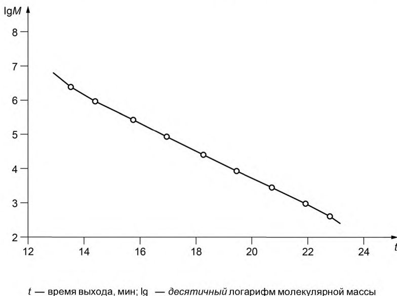
Рисунок 5 — Калибровочная кривая
